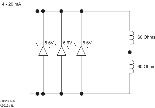
图 3. 等效电路
